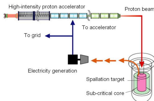
FIGURE 1.6: Schéma de principe du système hybride (source https://nsec.jaea.go.jp/ndre/ndre3/trans/objective-e.html ).
