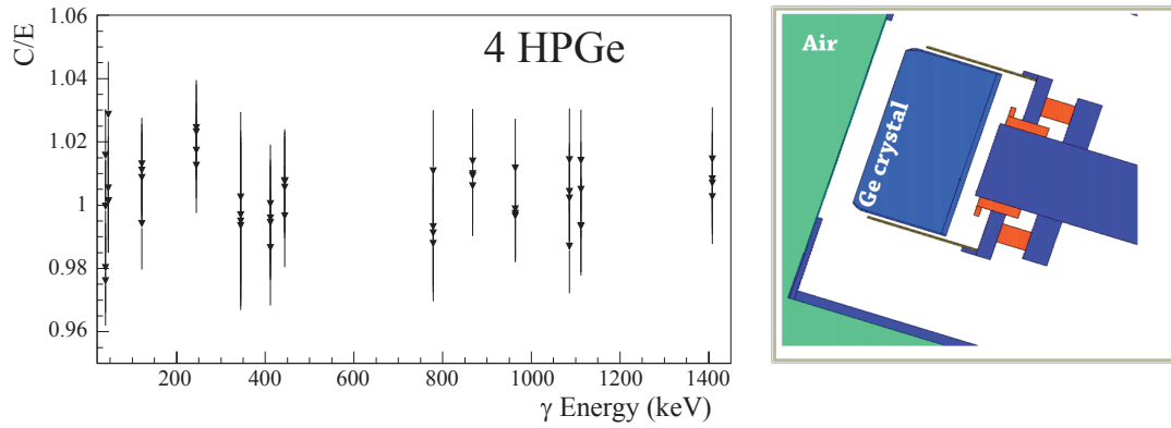
FIGURE 2.12: Rapport C/E (gauche) obtenu pour un détecteur après optimisation de sa géométrie (droite).
