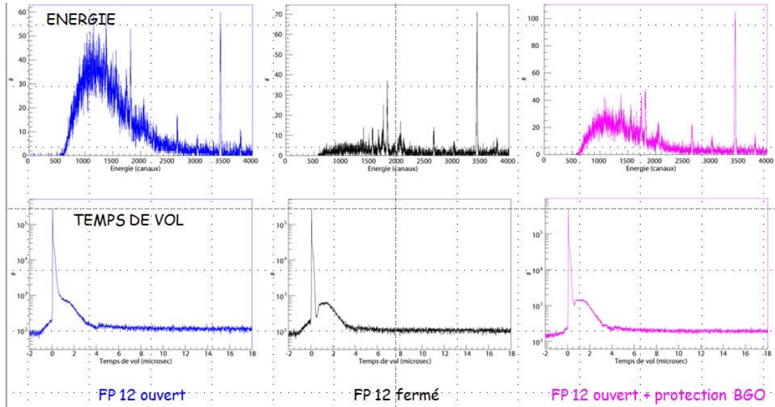
FIGURE 2.14: Mise en évidence de l'influence de l'environnement des autres bases de vol sur notre aire expérimentale (FP16/30 m) et de l'effet de protection d'un cristal BGO entourant le cristal de Germanium.
