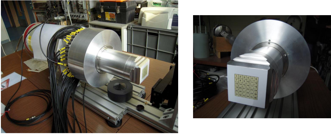
FIGURE 4.1: Photos du détecteur HPGe segmenté en 36 pixels sur son banc de test à l'IPHC (gauche) et zoom sur le capot du cristal (droite) et sa forme en escalier pour s'approcher au plus près de la cible sans intercepter le faisceau.
