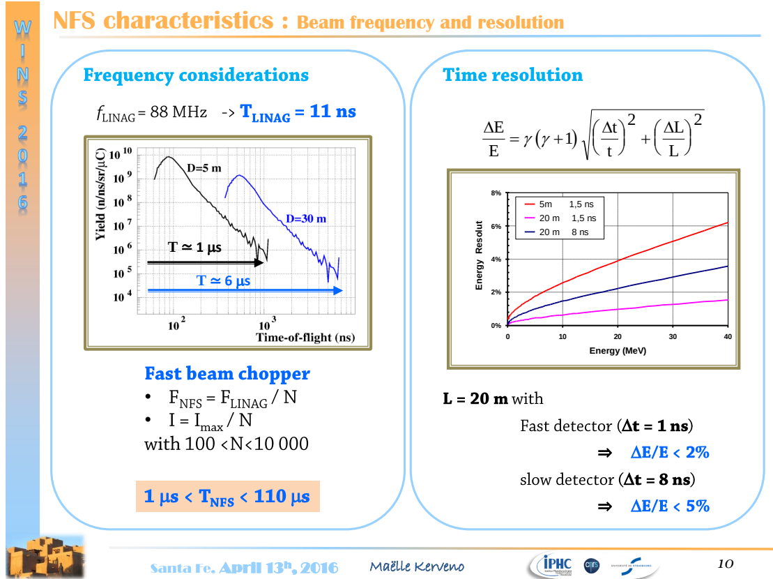
FIGURE 4.13: Fréquences du faisceau et résolutions en temps et en énergie accessibles à NFS.
