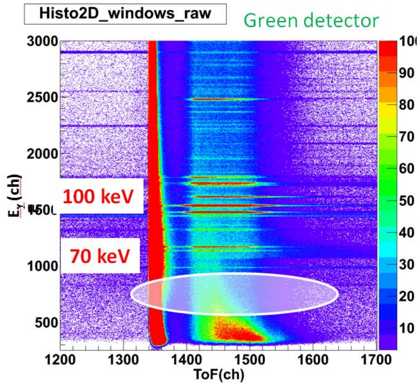
FIGURE 2.27: Spectre bi-dimensionnel de l'énergie \gamma en fonction du temps de détection pour le détecteur vert obtenu avec la cible d' ^{238}\text{U} . On voit clairement la contribution de \gamma -flash et les différentes transitions \gamma .
