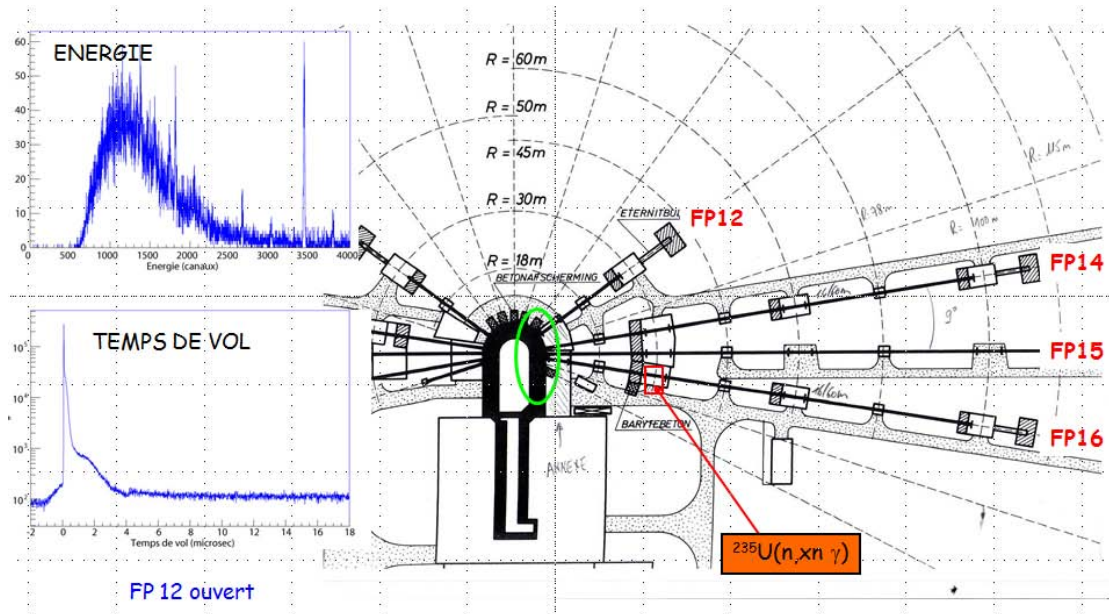
FIGURE 2.13: Environnement de notre aire expérimentale FP16/30 m et les spectres en énergie et en temps pour un détecteur Germanium obtenus avant la réduction du bruit de fond.
