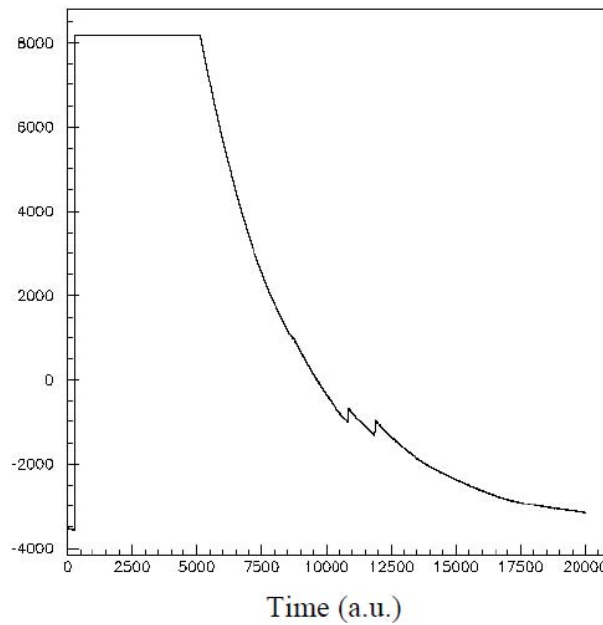
FIGURE 2.9: Exemple d'oscillogramme du signal à la sortie du pré-amplificateur enregistré lors de tests à n-TOF. La saturation correspond à une énergie d'environ 3.5 MeV et dure 75 \mu s.
