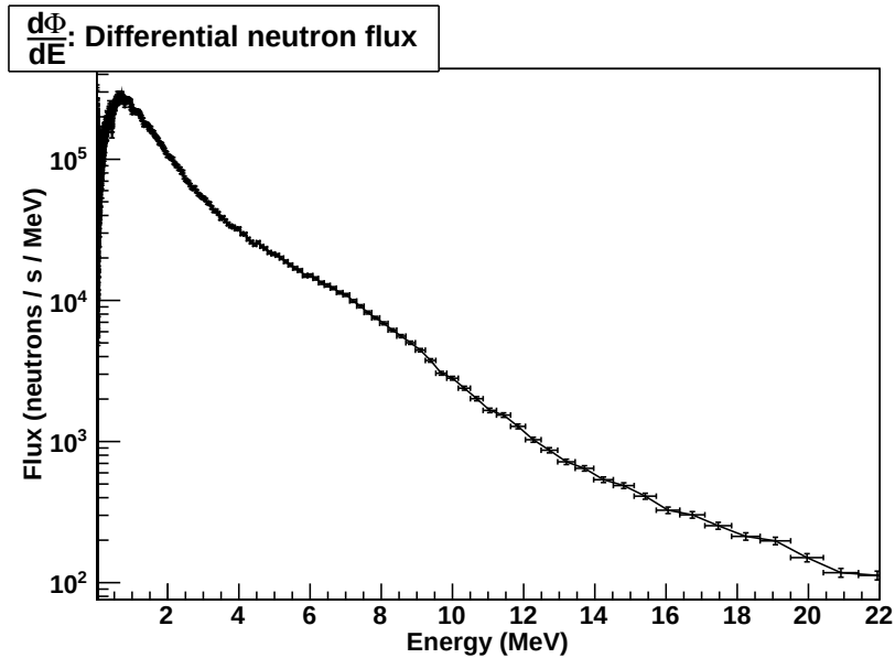
FIGURE 2.25: Flux de neutrons différentiel mesuré avec GRAPHME dans l'aire expérimentale FP16/30 m de GELINA.
