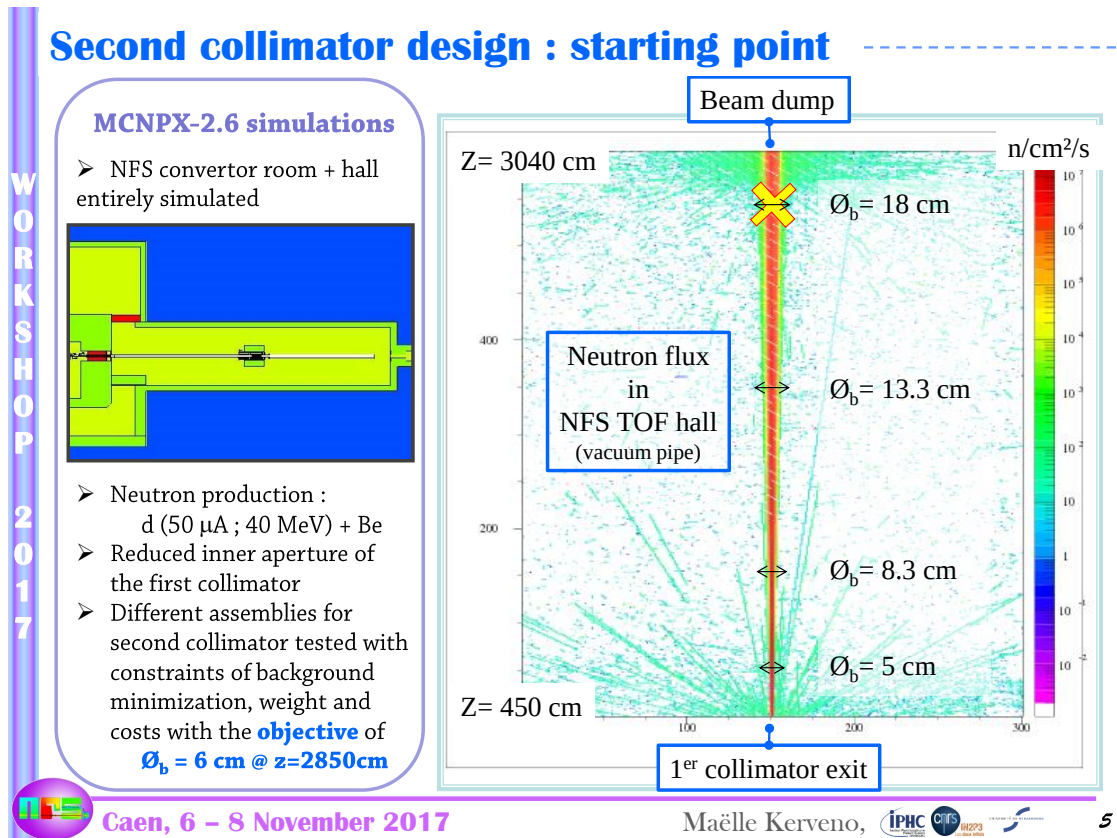
FIGURE 4.16: Simulation MCNPX-2.6 de la ligne sous vide du faisceau de neutrons (à droite). A gauche, définition des paramètres initiaux pour la simulation MCNPX-2.6 du second collimateur.
