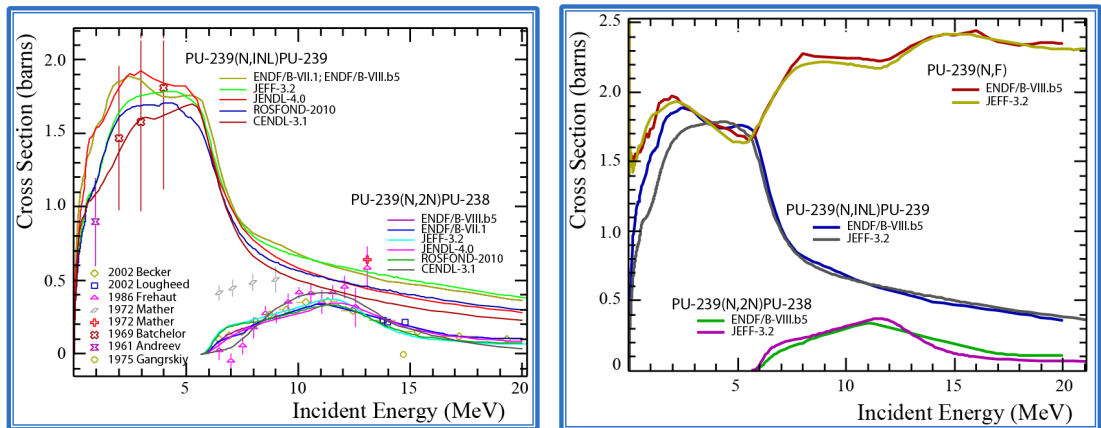
FIGURE 4.5: Droite : Sections efficaces évaluées (ENDF et HEFF) des différentes voies de réactions possibles sur ^{239}\text{Pu} , (n,f) , (n,n') et (n,2n) , entre 0 et 20 MeV. Gauche : Sections efficaces, évaluées et expérimentales, des réactions ^{239}\text{Pu}(n,n') et (n,2n) .
