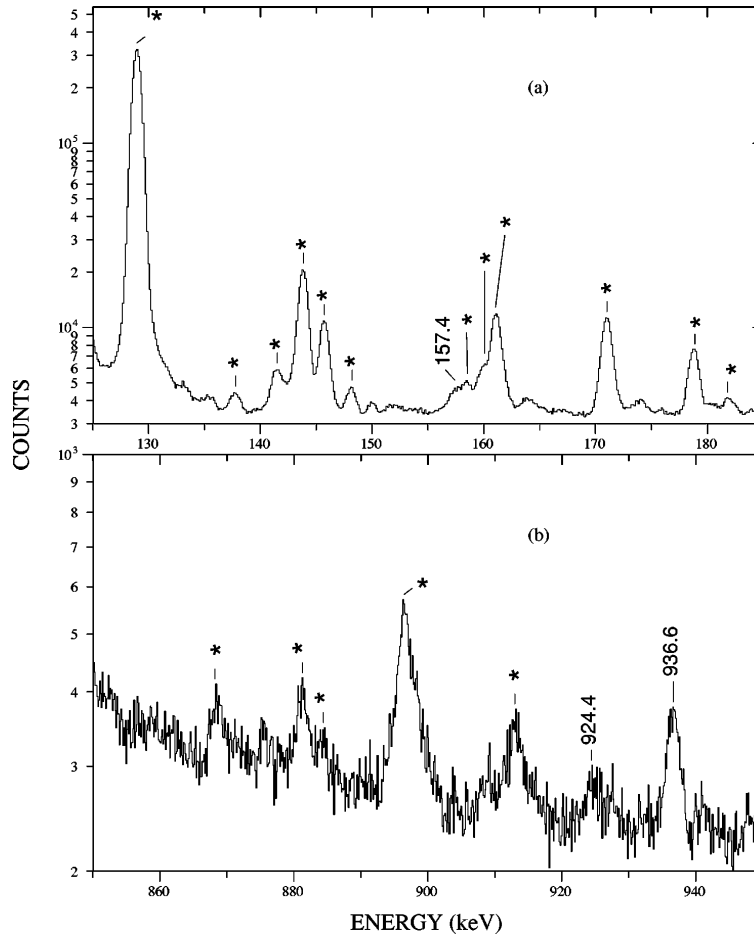
FIGURE 4.6: Distributions en énergie \gamma ( E_n = 11.35 MeV obtenues lors de la campagne GEANIE). Les pics marqués d'une étoile correspondent à la radioactivité et ceux des transitions \gamma dans ^{238}\text{Pu} sont repérés par leur énergie.
