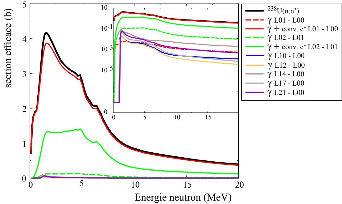
FIGURE 3.2: Section efficace totale ^{238}\text{U}(n, n') comparée aux contributions des sections efficaces ^{238}(n, n' \gamma) pour les transitions \gamma rejoignant le fondamental et la transition entre le deuxième et premier niveau. La correction de conversion interne est appliquée pour les transitions entre le premier niveau et le fondamental et le deuxième et le premier niveau. L'insert représente une vue logarithmique. Calculs réalisés avec le code de réaction nucléaire TALYS 1.8.
