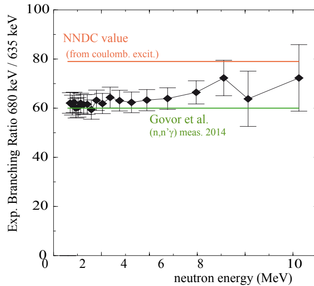
FIGURE 3.15: Rapport d'embranchement expérimental pour la décroissance du niveau 1^- à 680 keV de ^{238}\text{U} comparé au rapport d'embranchement présent dans NNDC et celui mesuré par Govor et al. .
