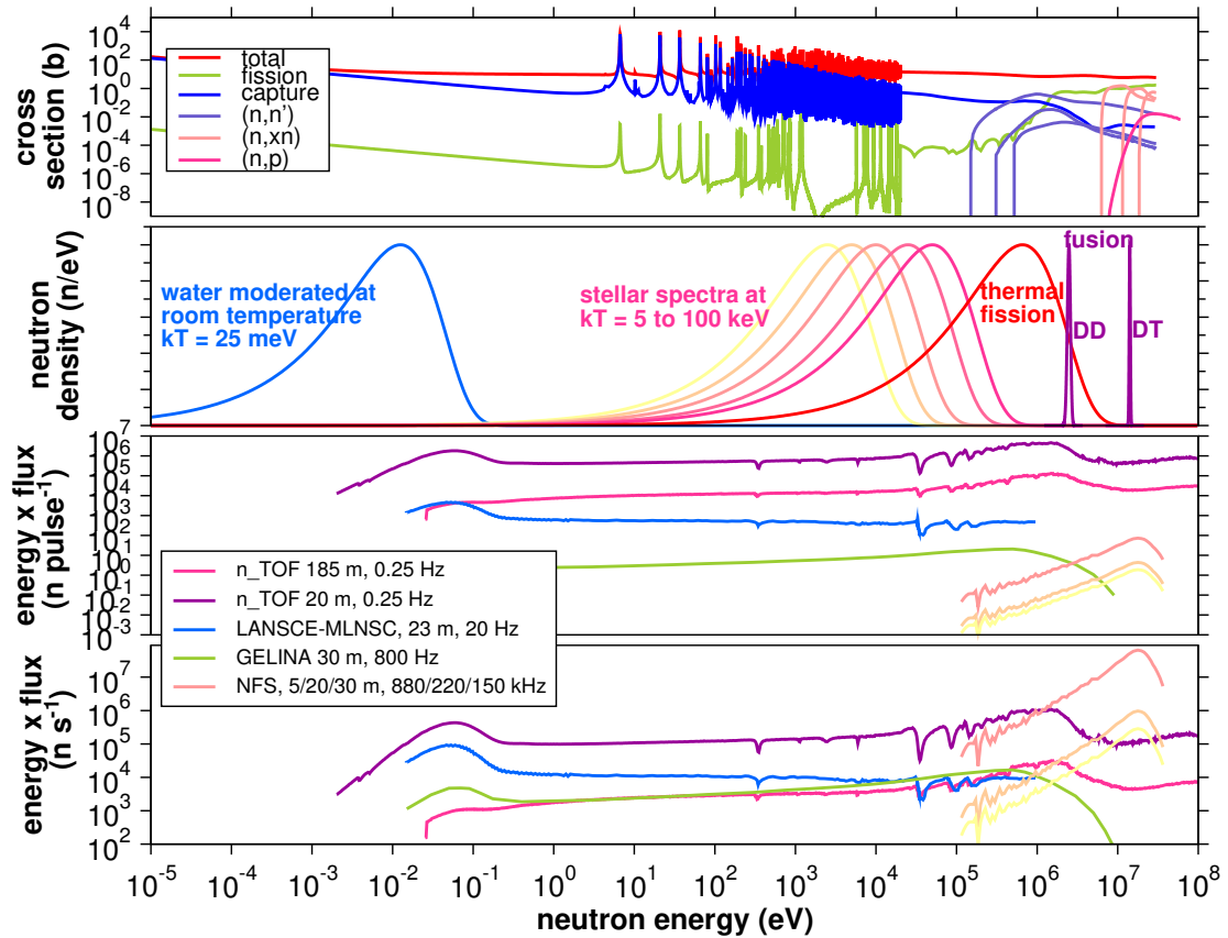
FIGURE 1.8: Comparaison des sections efficaces neutroniques sur l' ^{238}\text{U} et des spectres de neutrons typiques (haut), aux différents flux instantanés (milieu) et moyen (bas) des principales installations temps de vol mondiales. figure Frank Gunsing.
