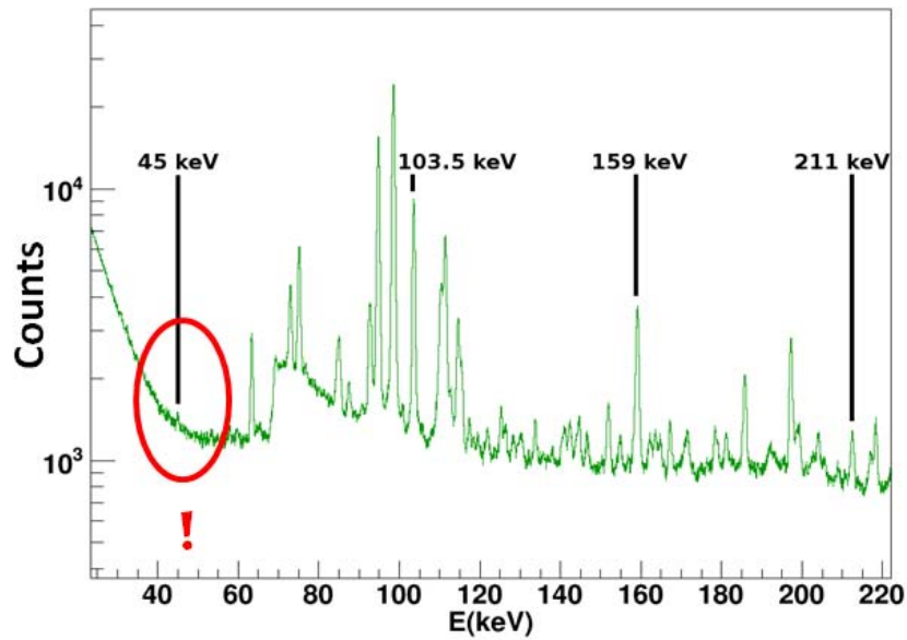
FIGURE 2.28: Portion de la distribution en énergie- \gamma , dans le cas de la réaction ^{238}\text{U}(n,n') , centrée sur les faibles énergies. On voit apparaître faiblement la transition à 45 keV ( 2^+-0^+ ) par rapport aux transitions provenant des niveaux supérieurs de la bande du fondamental.
