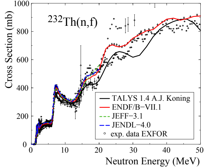
FIGURE 3.9: Section efficace de fission du Thorium 232 expérimentale, évaluée et calculée par TALYS-1.4.
