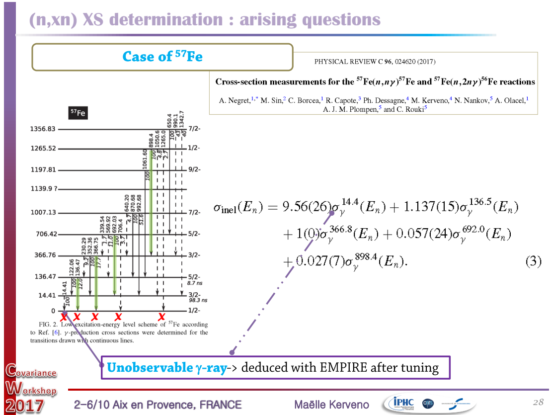
FIGURE 3.17: Portion du schéma de niveau du ^{57}\text{Fe} (gauche). Les transitions en trait plein sont celles qui ont pu être mesurées. Les croix rouges représentent les transitions qui atteignent l'état fondamental et qui doivent être utilisées pour reconstruire la section efficace inélastique totale. Les transitions surlignées en vert correspondent à celles effectivement utilisées pour ce calcul selon la formule à droite.
