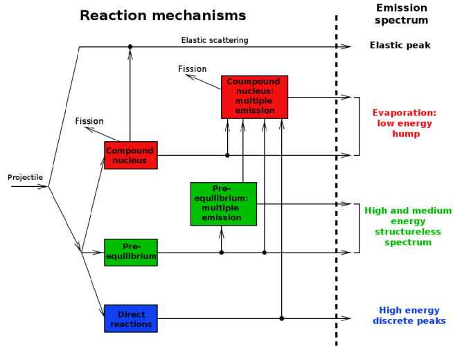
FIGURE 3.3: Schéma de la modélisation des réactions nucléaires.
