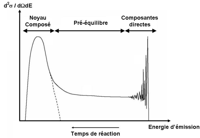
FIGURE 3.4: Spectre caractéristique de l'émission d'un neutron dans le domaine en énergie du continu.
