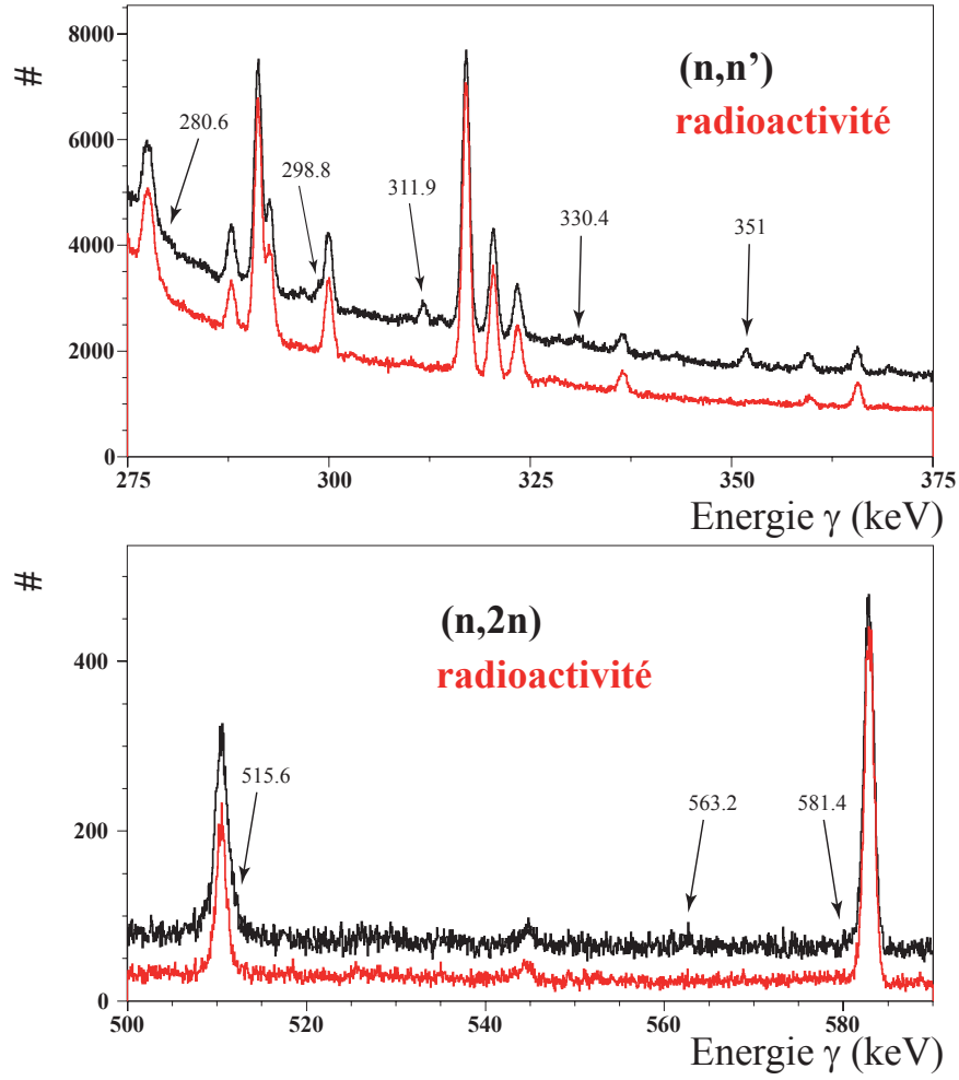
FIGURE 4.4: Portions du spectre \gamma enregistré avec 8 pixels du détecteur segmenté, pour une cible d' ^{233}\text{U} et après 867 heures de faisceau. Les différentes distributions correspondant à des fenêtres en temps relatives aux domaines de la radioactivité (rouge), des réactions (n,n') (noir-haut) et des réactions (n,2n) (noir-bas).
