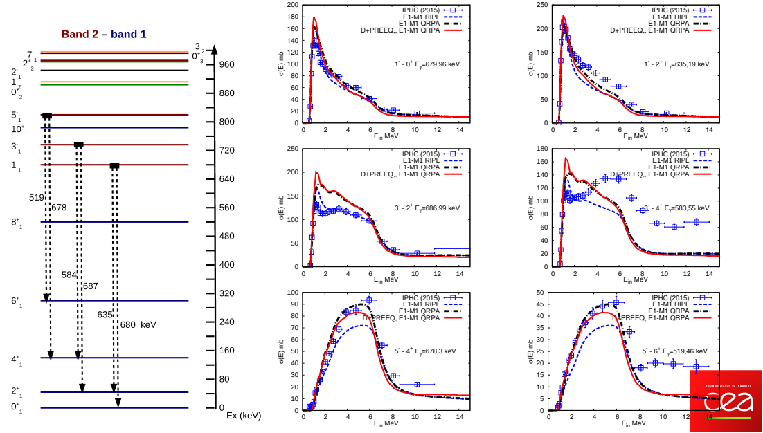
FIGURE 3.12: Sections efficaces ^{238}\text{U}(n, n' \gamma) expérimentales et calculées pour les transitions inter-bande (2-1). Trois approches pour les fonctions de force \gamma sont étudiées. La première (RIPL) décrit un calcul classique. E1-M1-QRPA est la combinaison d'un calcul classique avec une force \gamma microscopique et D+PREEQ, E1-M1 QRPA correspond à un calcul complet microscopique. Figure Marc Dupuis. Il faut noter que la transition à 584 keV ( 3^- - 4^+ ) est contaminée par une transition du plomb 208 à 583.19 keV à partir de 3 MeV.
