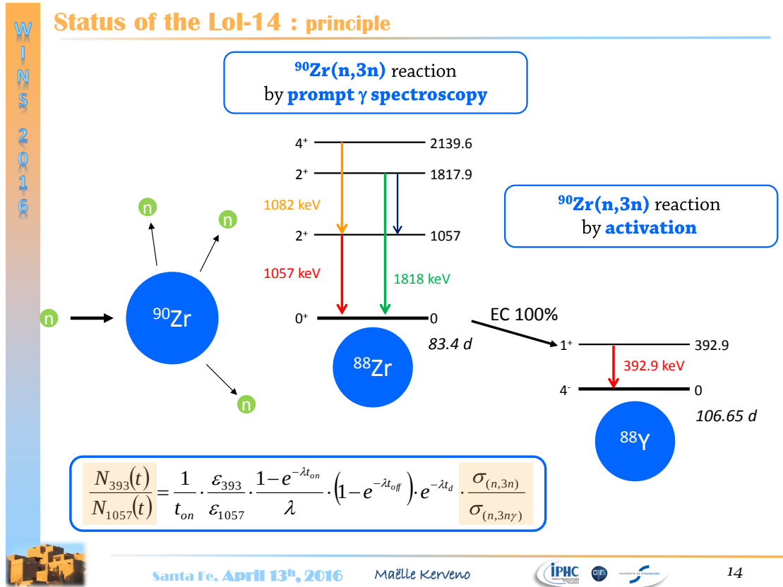
FIGURE 4.19: Schémas de niveaux partiels du ^{90}\text{Zr} et du ^{88}\text{Zr} produit par la réaction (n,3n) sur le ^{90}\text{Zr} et principe de la mesure simultanée de la section efficace ^{90}\text{Zr}(n,3n) par deux méthodes expérimentales différentes : la spectroscopie \gamma prompte et l'activation.
