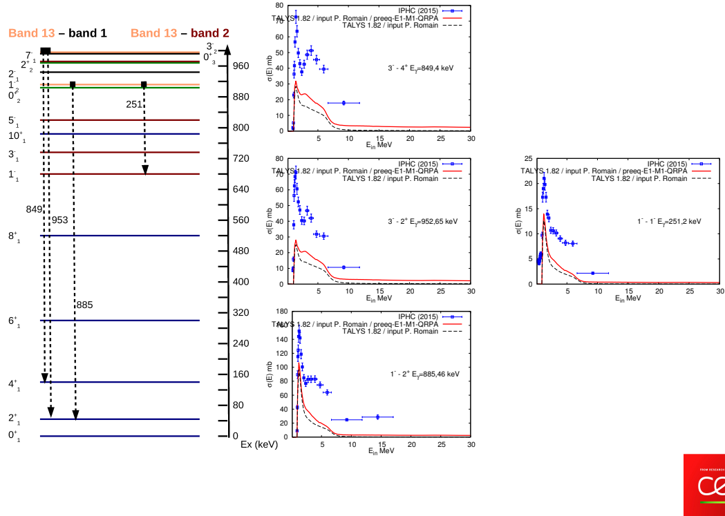
FIGURE 3.14: Sections efficaces ^{238}\text{U}(n, n' \gamma) expérimentales et calculées pour les transitions inter-bande (13-1 et 13-2). Deux approches pour les fonctions de force \gamma sont étudiées. la première décrit un calcul classique (Input P.romain) et preeq-E1-M1-QRPA correspond à un calcul complet microscopique. Figure Marc Dupuis.
