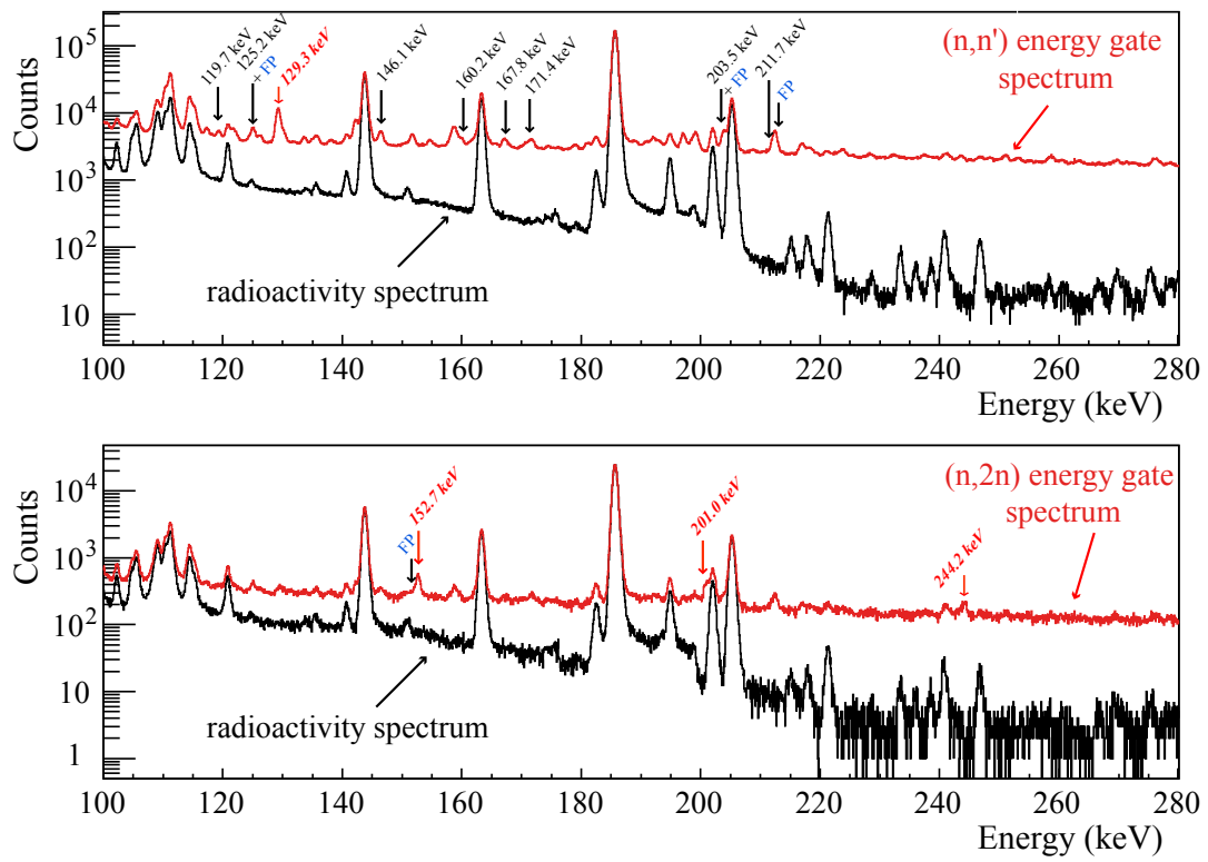
FIGURE 3.6: Portion du spectre en énergie \gamma pour des fenêtres en temps correspondant aux réactions (n,n') ((a), rouge) et (n,2n) ((b), rouge) comparée au spectre de décroissance radioactive (noir) pour la cible ^{235}\text{U} . Les transitions analysées sont repérées en italique et en rouge, les transitions provenant de la décroissance des produits de fission sont labellisées "FP" en bleu.
