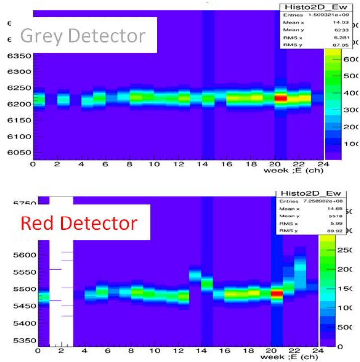
FIGURE 2.23: Suivi de la position (en canal) du pic à 511 keV en fonction des semaines de prise de données pour le détecteur vert et rouge.
