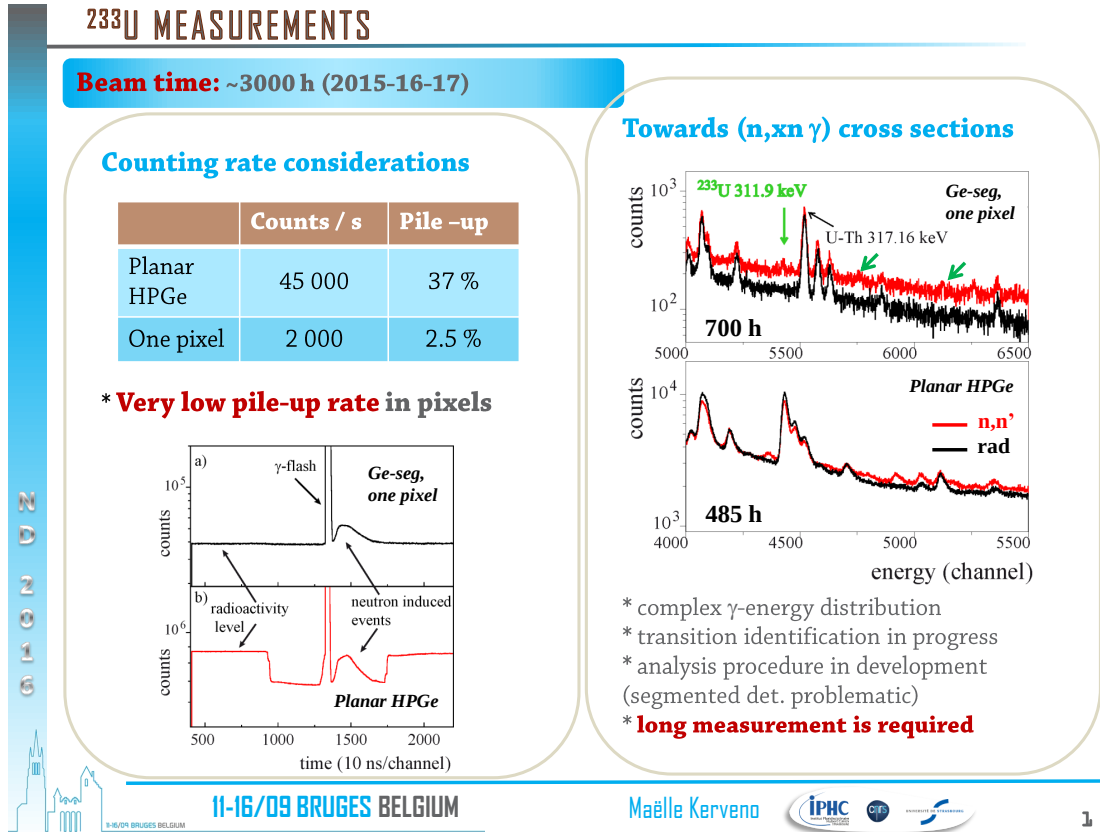
FIGURE 4.2: Illustration du gain obtenu avec le détecteur segmenté, dans le cas de l'utilisation de cibles très radioactives (ici ^{233}\text{U} ), concernant le taux d'empilement et la résolution en énergie. Extrait de la présentation fait à la conférence ND2016, Bruges, Belgique.
