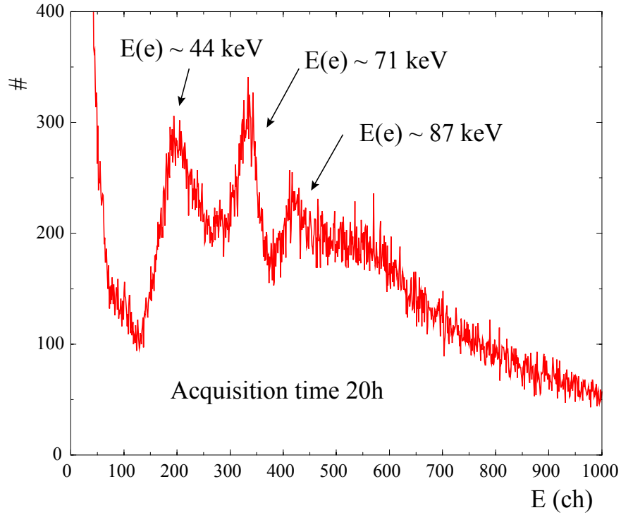
FIGURE 4.10: Distribution en énergie, issue de la radioactivité de l'échantillon d'uranium, mesurée pendant 20 h de temps d'acquisition.
