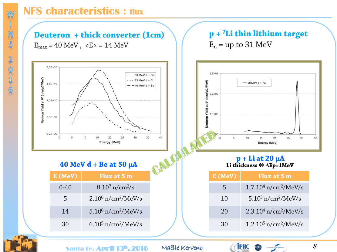
FIGURE 4.12: Caractéristiques des différents faisceaux de neutrons pouvant être produits à NFS.
