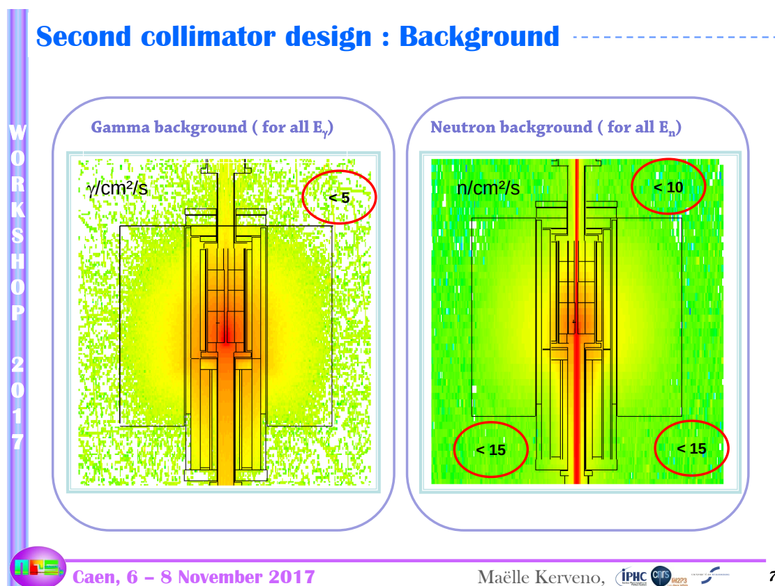
FIGURE 4.18: Simulation du bruit de fond \gamma (à gauche) et neutrons (à droite) dans et aux alentours du second collimateur.
