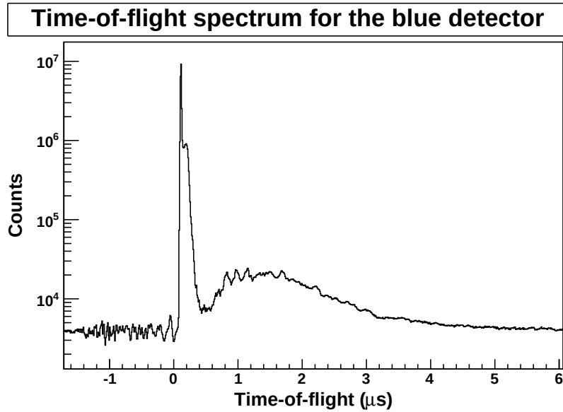
FIGURE 2.16: Distribution en temps d'un détecteur Germanium affectée par des oscillations dues au rayonnement électromagnétique généré par les klystrons de GELINA.
