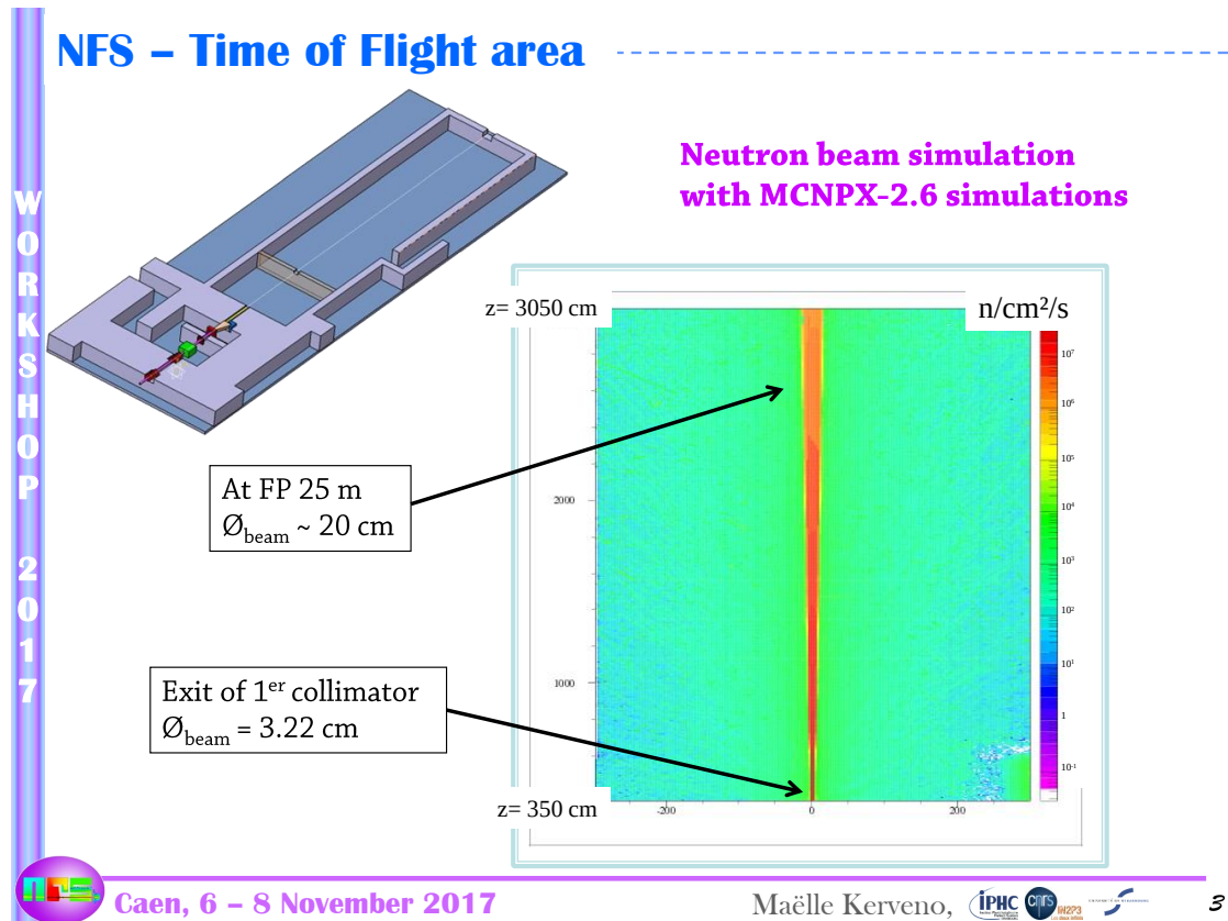
FIGURE 4.14: Simulation MCNPX-2.6 du faisceau de neutrons de l'installation NFS, de la sortie du premier collimateur ( z=350 \text{ cm} ) et tout au long de la salle de temps de vol.
