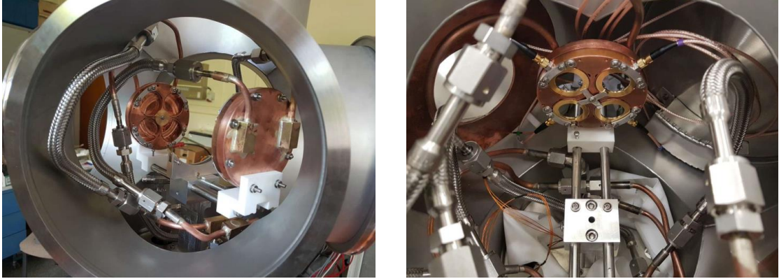
FIGURE 4.9: Photo de l'intérieur de la chambre de DELCO avec les supports des détecteurs (gauche) et les détecteurs insérés (droite).
