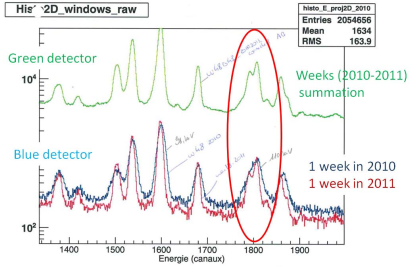
FIGURE 2.24: Portion des distributions en énergie \gamma pour le détecteur VERT (ligne verte) pour un lot de plusieurs semaines sommées et pour le détecteur BLEU pour deux semaines distinctes de 2010 (ligne bleue) et de 2011 (ligne rouge). On voit la perte de résolution sur le lot de 2010 pour les pics présents autour du canal 1800.
