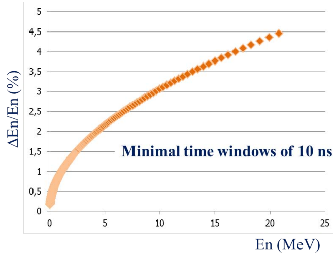
FIGURE 2.10: Evolution de la résolution en énergie neutron en fonction de l'énergie neutron à 30 m de la source de production.
