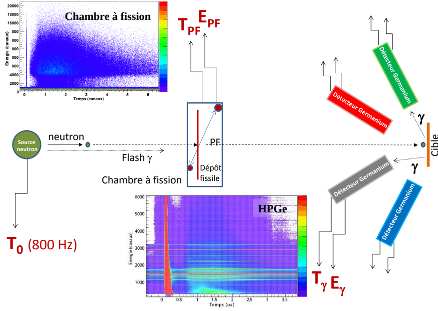
FIGURE 2.8: Schéma de principe du système de détection pour la méthode de la spectroscopie \gamma prompt couplée à des mesures de temps de vol. Le schéma n'est pas à l'échelle et ne respecte pas les proportions.
