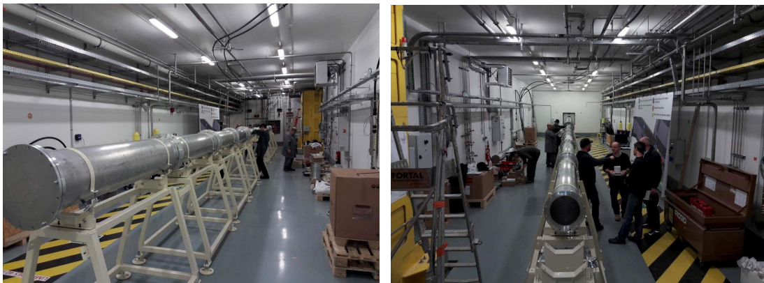
FIGURE 4.15: Photos de la ligne faisceau, conçue et construite à l'IPHC, une fois installée dans la salle temps de vol de NFS.
