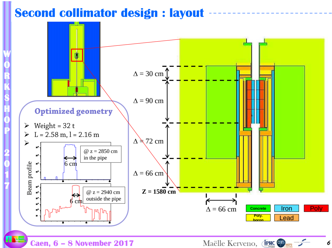
FIGURE 4.17: Schéma du second collimateur et de son blindage tels qu'ils sont simulés avec MCNPX-2.6. L'encart en bas à gauche montre le profil du faisceau obtenu alors à une distance de 28.5 m de la source de neutrons et juste après la fin de la ligne sous vide.
