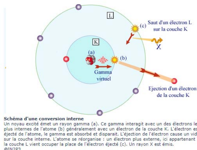
FIGURE 4.7: Principe de la conversion interne. Source http://www.laradioactivite.com .
