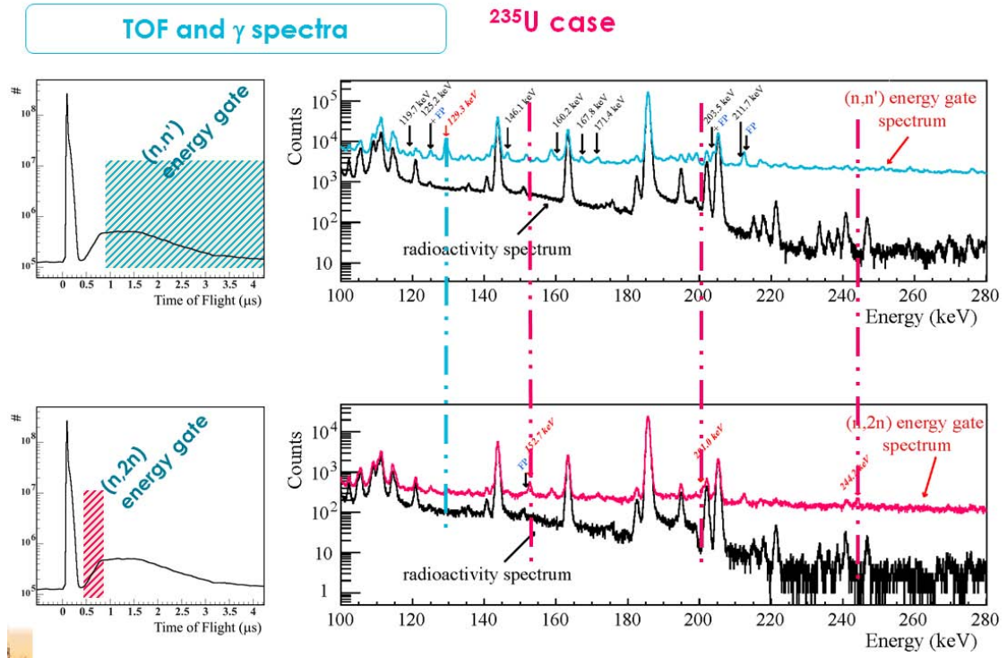
FIGURE 2.26: Illustration de la génération des distributions en énergie \gamma (spectres de droite) à partir des fenêtres en temps appliquées sur la distribution en temps (spectres de gauche) obtenues pour les données de l' ^{235}\text{U} .
