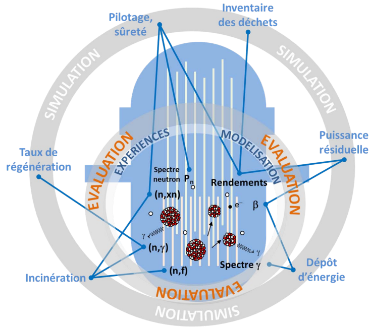
FIGURE 1.11: Schéma résumant le cycle de l'évaluation dans le cadre des données nucléaires pour les réacteurs et dans lequel le projet NACRE s'inscrit.
