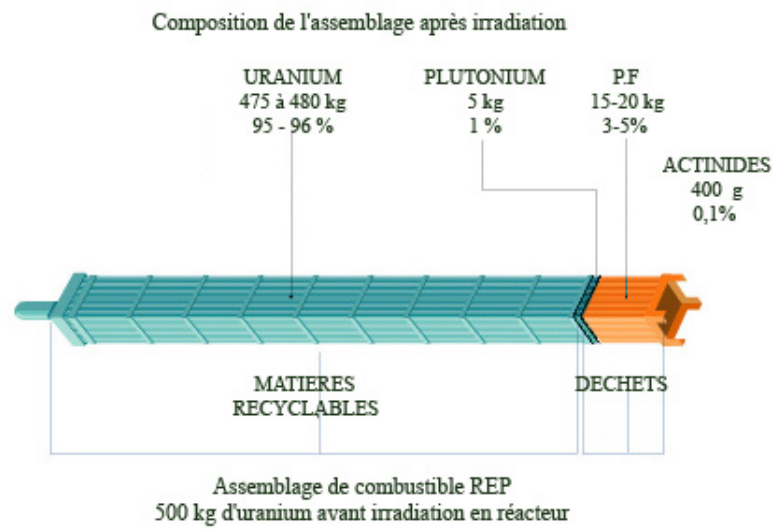
FIGURE 1.4: Composition d'un assemblage après irradiation dans un REP (initialement 500 kg d'uranium étaient présents).
