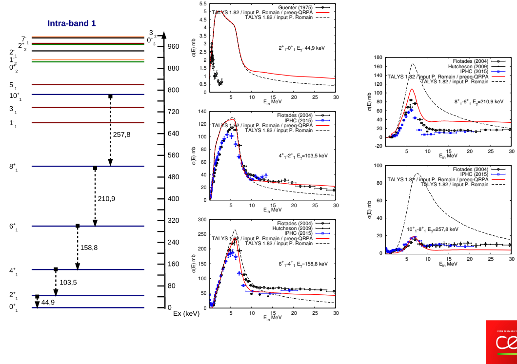
FIGURE 3.10: Sections efficaces ^{238}\text{U}(n, n' \gamma) expérimentales et calculées pour les transitions dans la bande du fondamental. La différence entre le calcul microscopique (QRPA) ou classique (excitons) pour le pré-équilibre est clairement visible sur les transitions au delà du spin 4\hbar . Figure Marc Dupuis.
