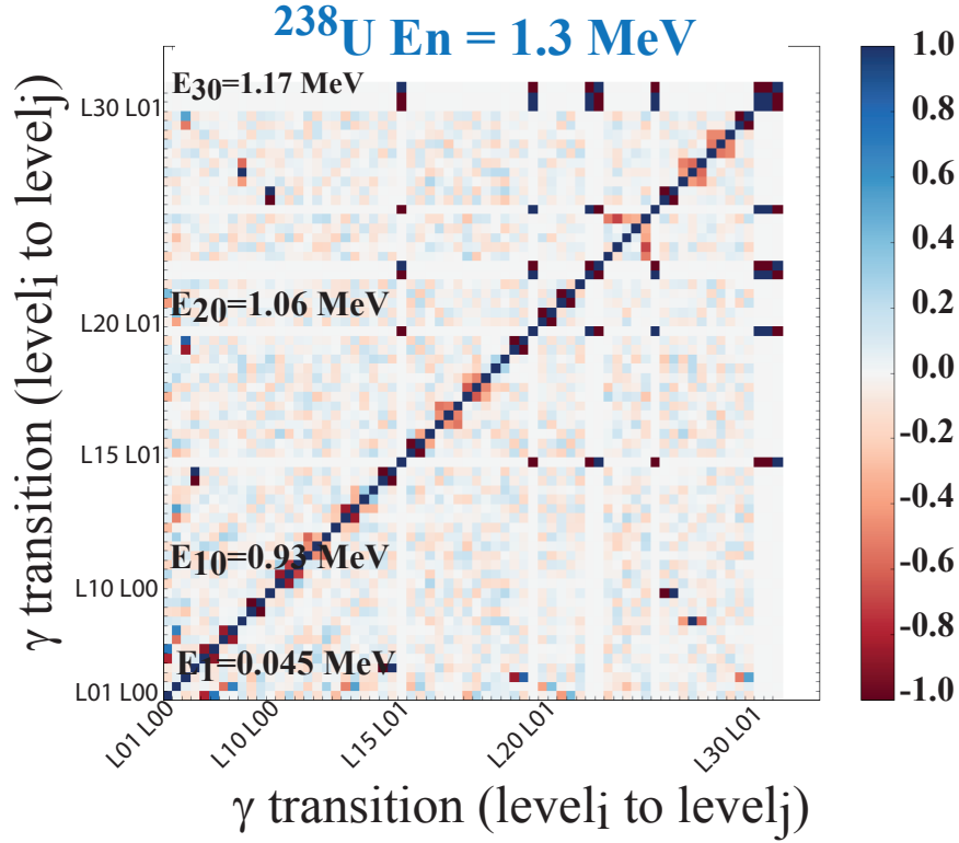
FIGURE 3.19: Matrice de corrélation des sections efficaces de transition \gamma lors de réactions ^{238}\text{U}(n,n') et pour une énergie incidente de 1.3 MeV. Les sections efficaces ont été obtenues via une simulation Monte Carlo avec le code TALYS en faisant varier les rapports d'embranchement dans la structure de ^{238}\text{U} aléatoirement.
