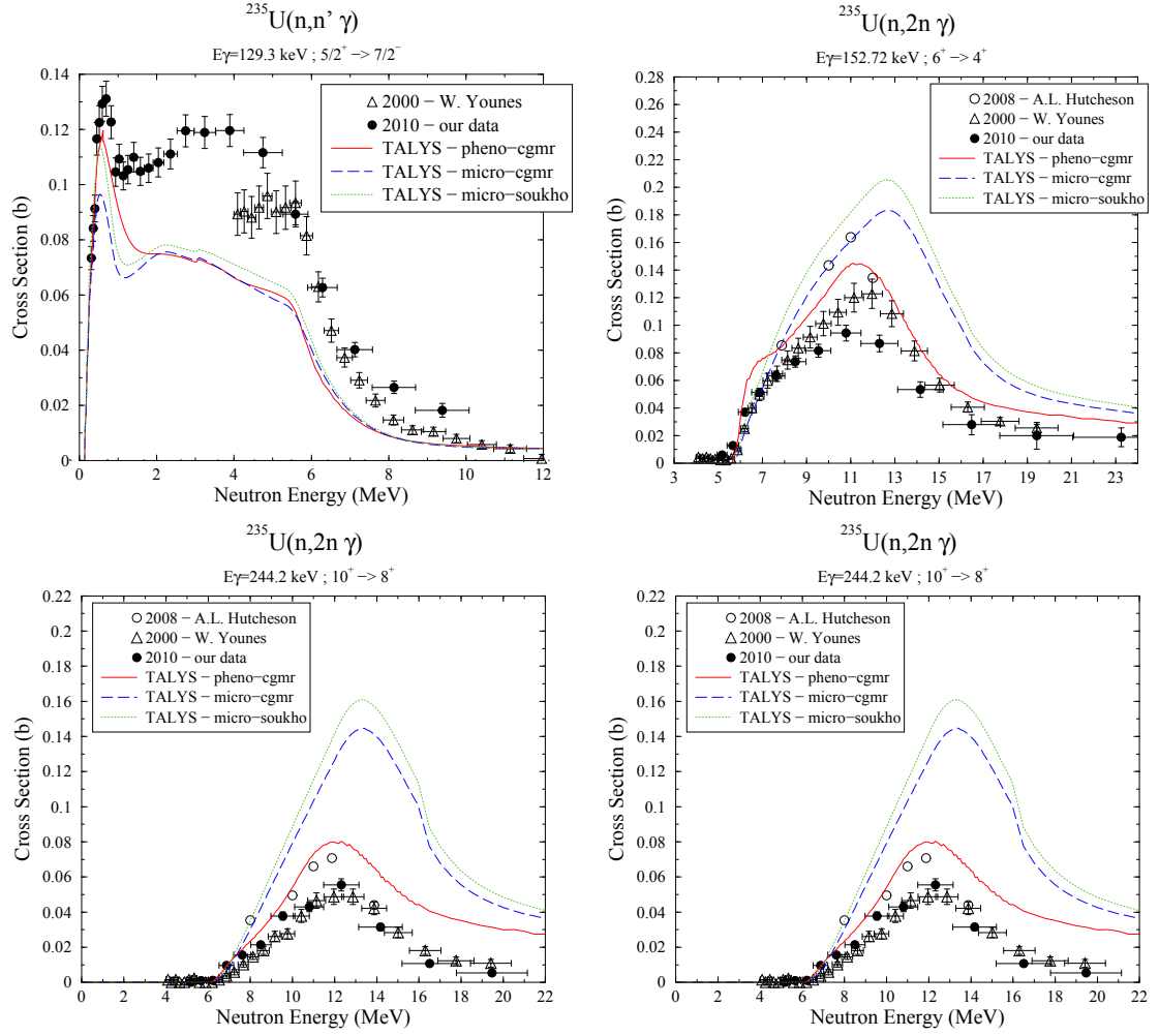
FIGURE 3.7: Sections efficaces ^{235}\text{U}(n, n' \gamma) et ^{235}\text{U}(n, 2n \gamma) comparées aux données expérimentales existantes et aux prédictions du code TALYS avec différents modèles et paramètres d'entrée.
