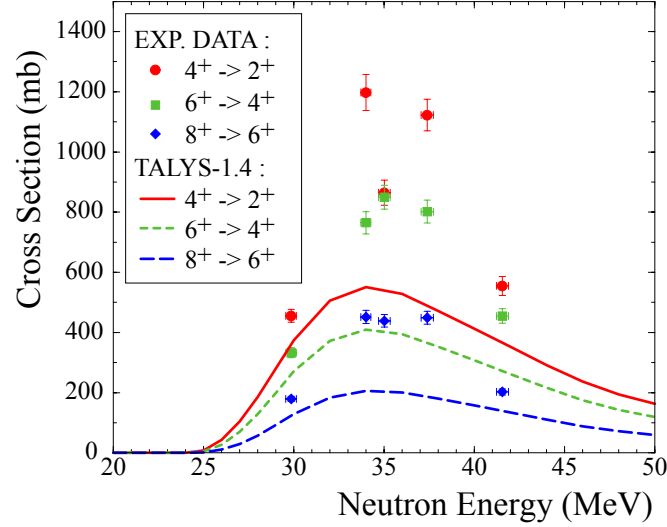
FIGURE 3.8: Sections efficaces ^{232}\text{Th}(n, 5n \gamma) pour trois transitions de la bande du fondamentale du ^{228}\text{Th} comparées aux prédictions du code TALYS-1.4 (calculs réalisés par A.J. Koning).
