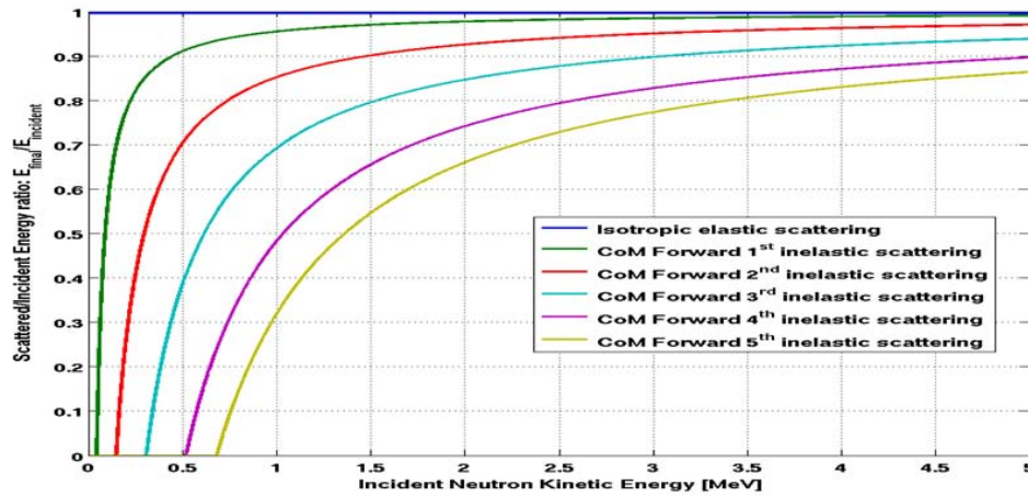
FIGURE 2.1: Rapport énergie finale sur énergie initiale en fonction de l'énergie incidente du neutron pour les chocs élastiques et inélastiques.
