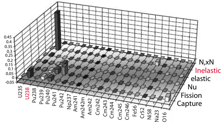
FIGURE 2.4: Contribution des incertitudes sur les sections efficaces des réactions à l'incertitude sur le k_{\text{eff}} du système EFR et ce pour 21 isotopes.
