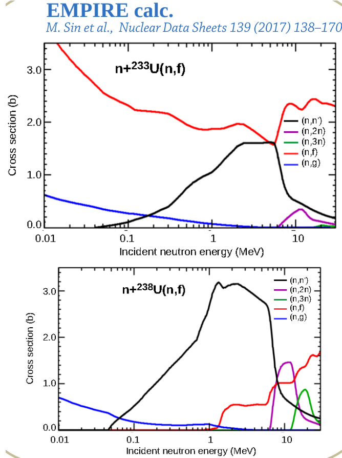
FIGURE 4.3: Sections efficaces des différentes voies de réactions possibles entre 0 et 30 MeV calculées par le code de réaction nucléaire EMPIRE pour l'uranium 233 et 238.
