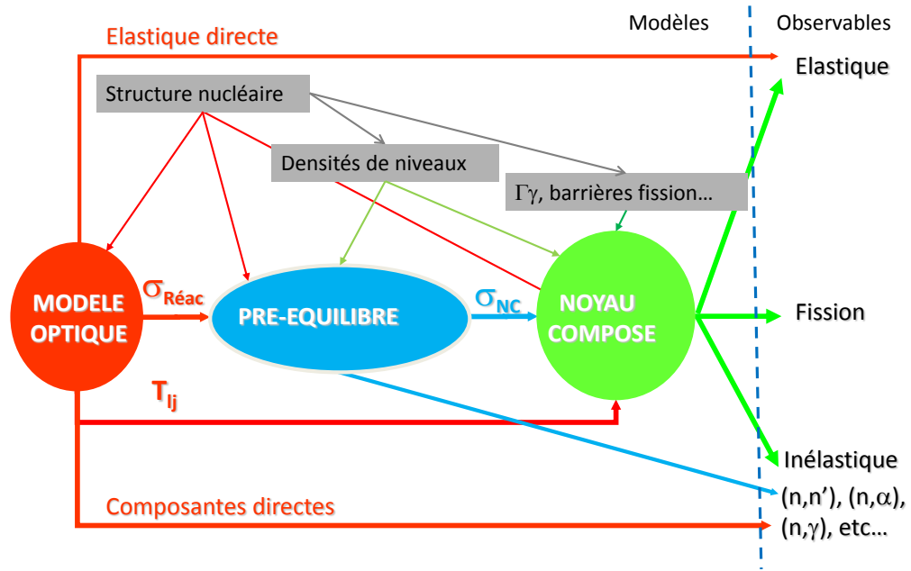
FIGURE 3.5: Exemple d'enchâinement des modèles tels qu'ils sont implémentés dans le code de réaction nucléaire TALYS.
