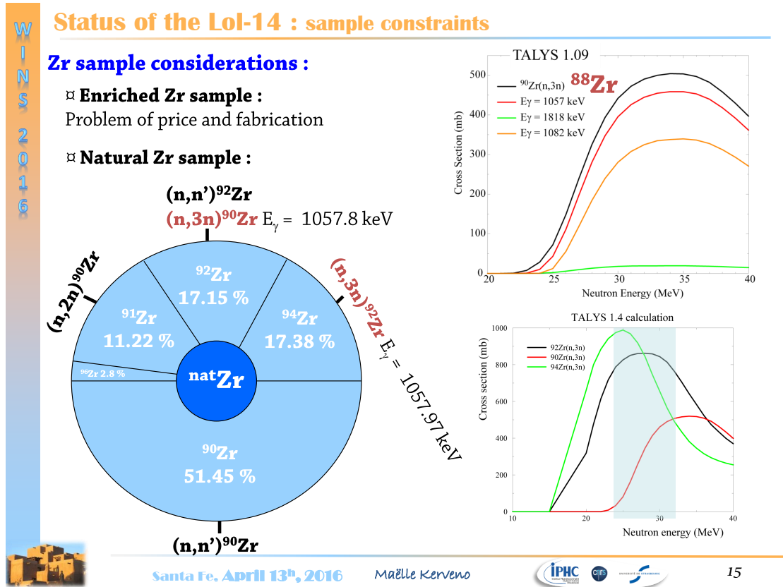
FIGURE 4.20: Contraintes de l'expérience liées à la composition d'une cible de Zr naturel (à gauche). À droite, différentes sections efficaces totales (n,xn) sur les principaux isotopes du Zr, et partielles (n,xn \gamma ) pour le ^{90}\text{Zr} , calculées par le code TALYS.
