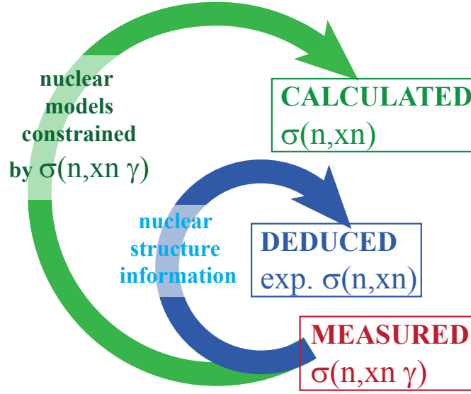
FIGURE 3.1: Schéma des deux stratégies possibles pour déduire les sections efficaces (n,xn) totales des sections efficaces (n,xn \gamma) mesurées.
