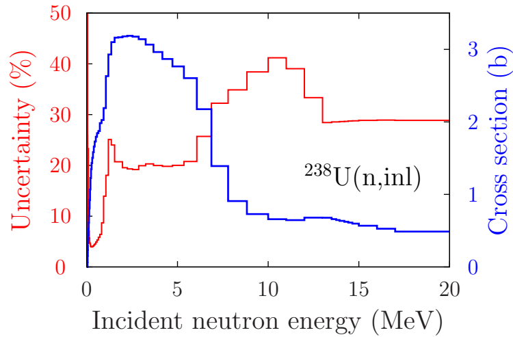
FIGURE 2.3: Section efficace de diffusion inélastique sur ^{238}\text{U} provenant de la base de données ENDF/B-VII.1. L'ordonnée à gauche correspond aux incertitudes et l'ordonnée à droite à la section efficace.
