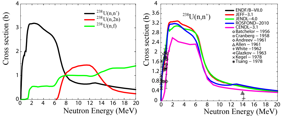
FIGURE 2.2: Section efficace de diffusion inélastique, de fission et de réaction (n,2n) sur ^{238}\text{U} (gauche) et comparaison des bases de données expérimentales aux bases de données évaluées.
