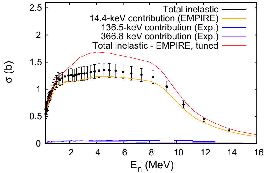
FIGURE 3.18: Section efficace inélastique totale pour le ^{57}\text{Fe} obtenue avec une combinaison de données expérimentales et modélisées par le code EMPIRE. Les contributions de deux autres niveaux sont montrées.
