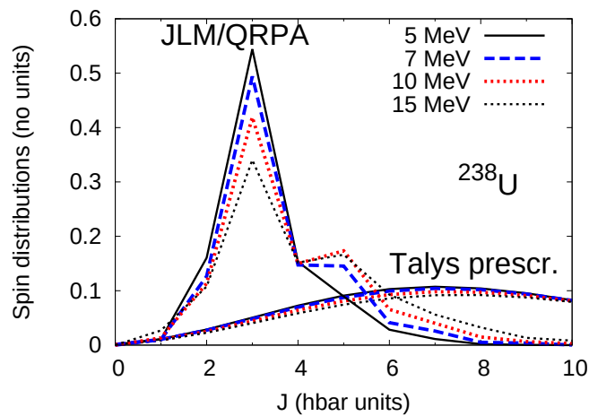
FIGURE 3.11: Distributions en spin du noyau résiduel formé après l'émission de pré-équilibre d'un neutron, pour la réaction n + ^{238}\text{U} , obtenues avec un calcul microscopique (JLM/QRPA) par rapport à un calcul classique d'excitons (Talys Prescr.).
