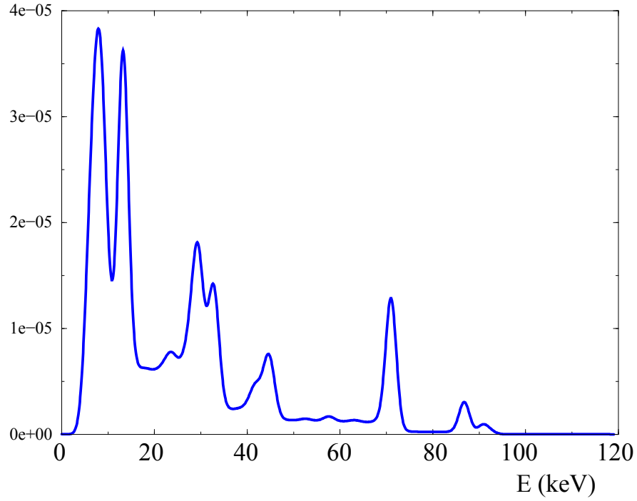
FIGURE 4.8: Distribution en énergie des principaux électrons et photons issus de la radioactivité de l'uranium 238 simulée avec MCNPX.
