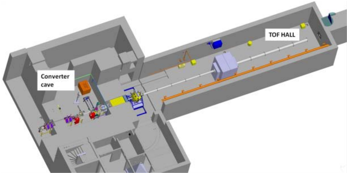
FIGURE 4.11: Schéma de l'installation NFS où les salles du convertisseur et du temps de vol sont visibles.
