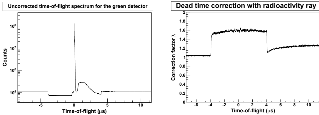
FIGURE 2.11: A gauche : Spectre temps de vol obtenu pour un détecteur Germanium où les événements "pile-up" ne sont pas considérés. A droite : le facteur de correction du temps mort et du "pile-up" en fonction du temps obtenu en suivant une raie de radioactivité.
