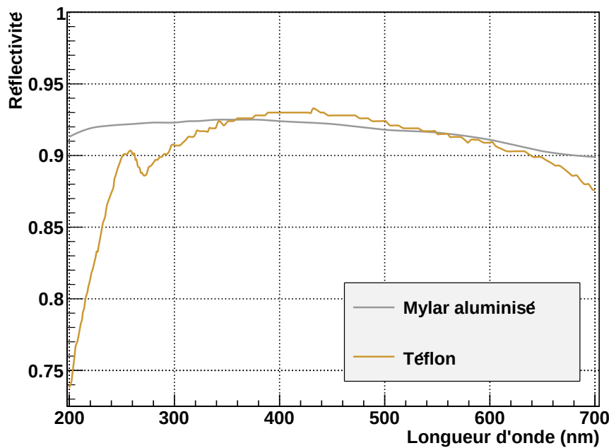
FIGURE 3.25 – Réflectivité mesurée en fonction de la longueur d'onde de la lumière pour le Mylar aluminisé et le Telfon.
