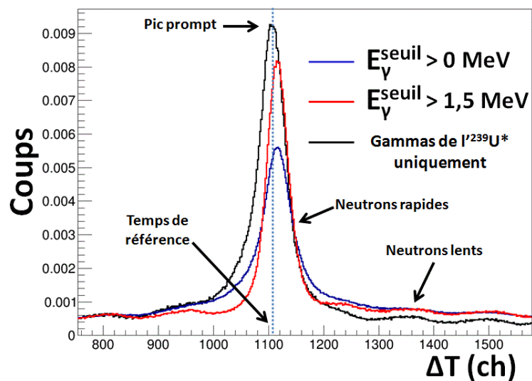
Figure D.19.: Proportion d'évènements détectés (normalisée à 1) en fonction de la différence en temps. La courbe noire ne concerne que les gammas émis par 1^{239}U^* d'énergie d'excitation inférieure au S_n , alors que les courbes rouge et bleue incluent également la contribution due aux neutrons détectés pour différents seuils de détection en énergie. Le temps de coïncidence de référence correspond au maximum du pic gamma prompt et est symbolé par la ligne en pointillée.
