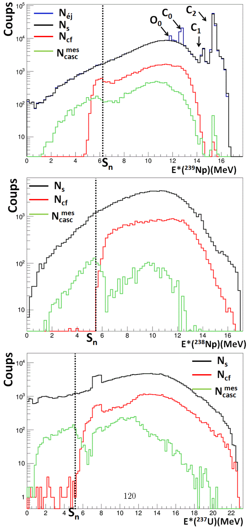
Figure D.27.: Spectres singles N_s(E^*) , de coïncidences fission N_{cf}(E^*) et de coïncidences gammas N_{\text{mes casc}}^{\text{mes}}(E^*) pour les noyaux composés ^{237}\text{U} , ^{238}\text{Np} et ^{239}\text{Np} . La ligne en pointillé représente l'énergie de séparation du neutron.
