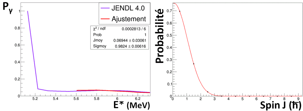
Figure E.24.: L'ajustement de P_\gamma^{JENDL} pour ^{237}\text{U}^* à partir de l'équation E.10 est représenté en rouge (à gauche). Distribution de spin obtenue grâce à l'ajustement de P_\gamma^{JENDL} sur la gamme énergétique [5,6-6,3 MeV] (à droite).
