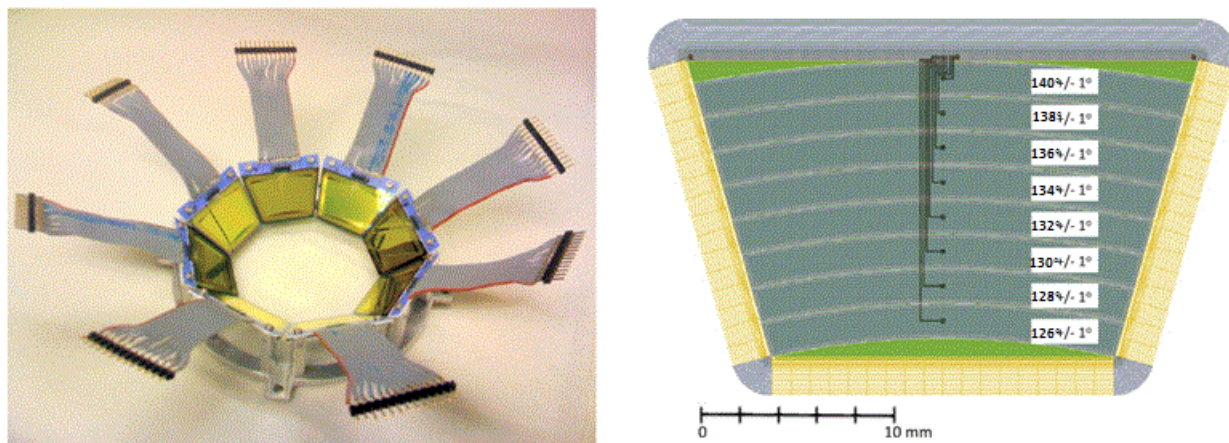
Figure C.5.: Détecteur SiRi avec connexions électroniques (à gauche). Vue schématisée d'un télescope de SiRi avec les huit pistes situées à des angles de 126^\circ à 140^\circ par rapport à l'axe du faisceau (à droite).
