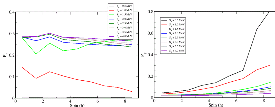
Figure E.36.: Probabilités de fission (à gauche) et d'émission gamma (à droite) de l' ^{237}\text{U}^* en fonction du spin à différentes E^* pour un moment d'inertie décrit par le modèle du rotateur rigide. Calculs réalisés par le code FIFRELIN.
