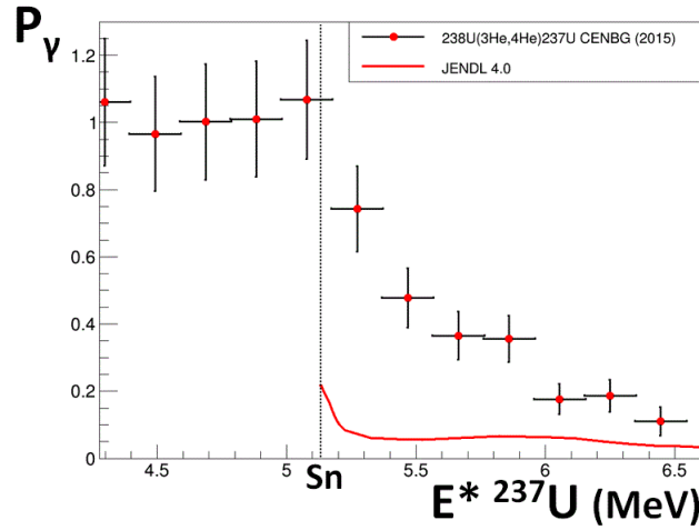
Figure E.21.: Probabilité d'émission gamma de l^{237}\text{U}^* en fonction de l'énergie d'excitation comparée à l'évaluation JENDL 4.0.
