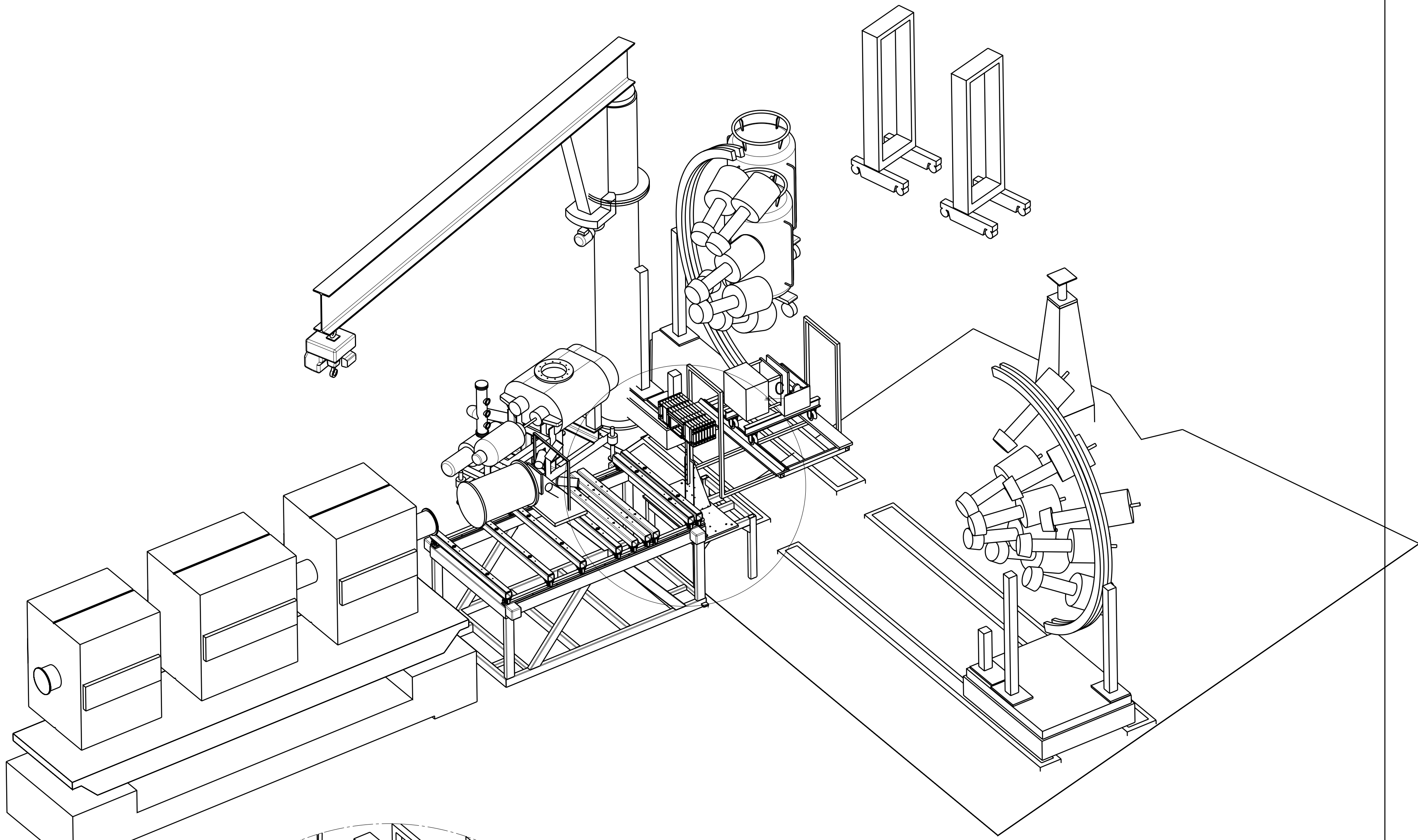
Vue isométrique Echelle : 1:30
