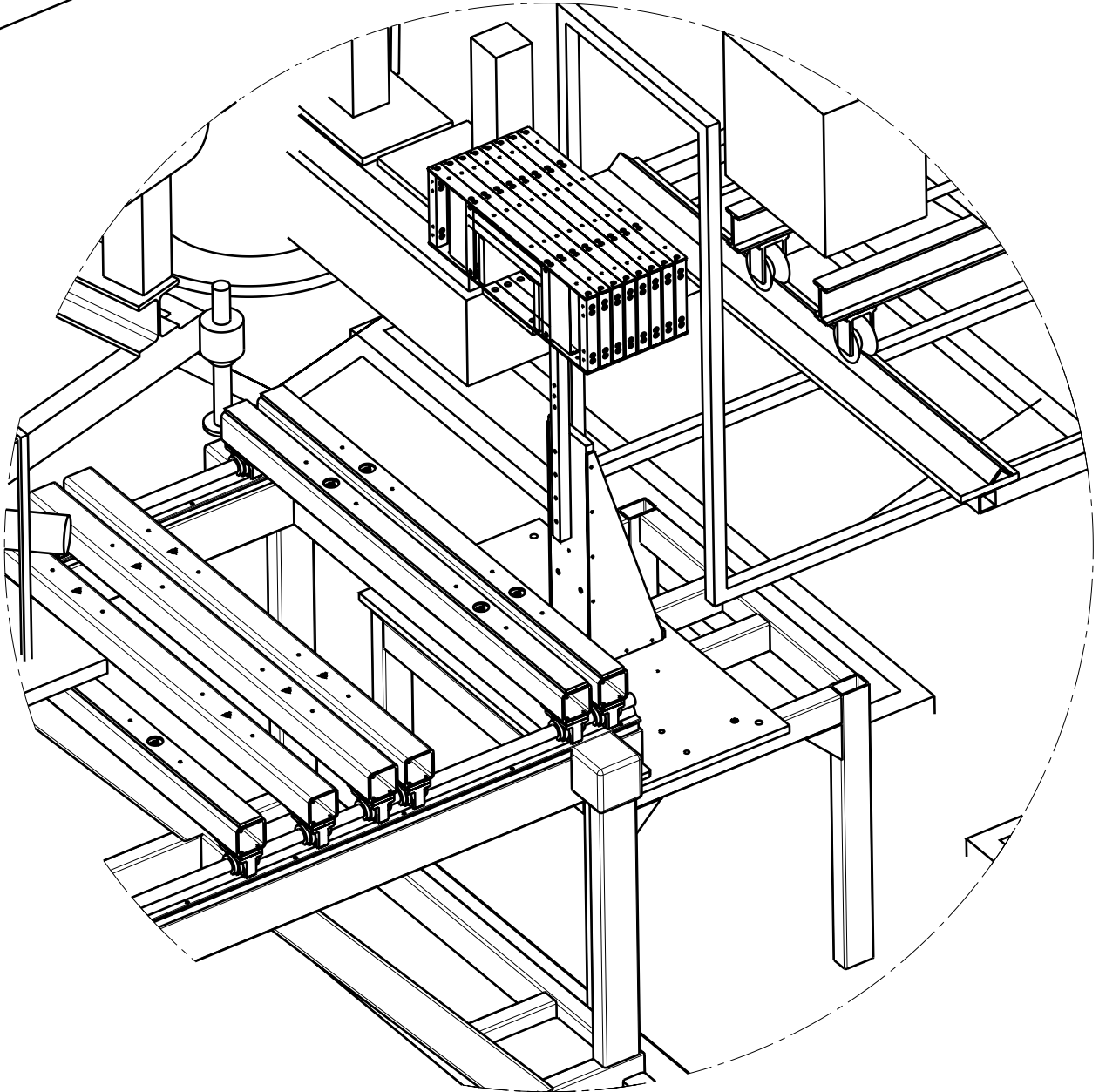
Détail C Echelle : 1:15
