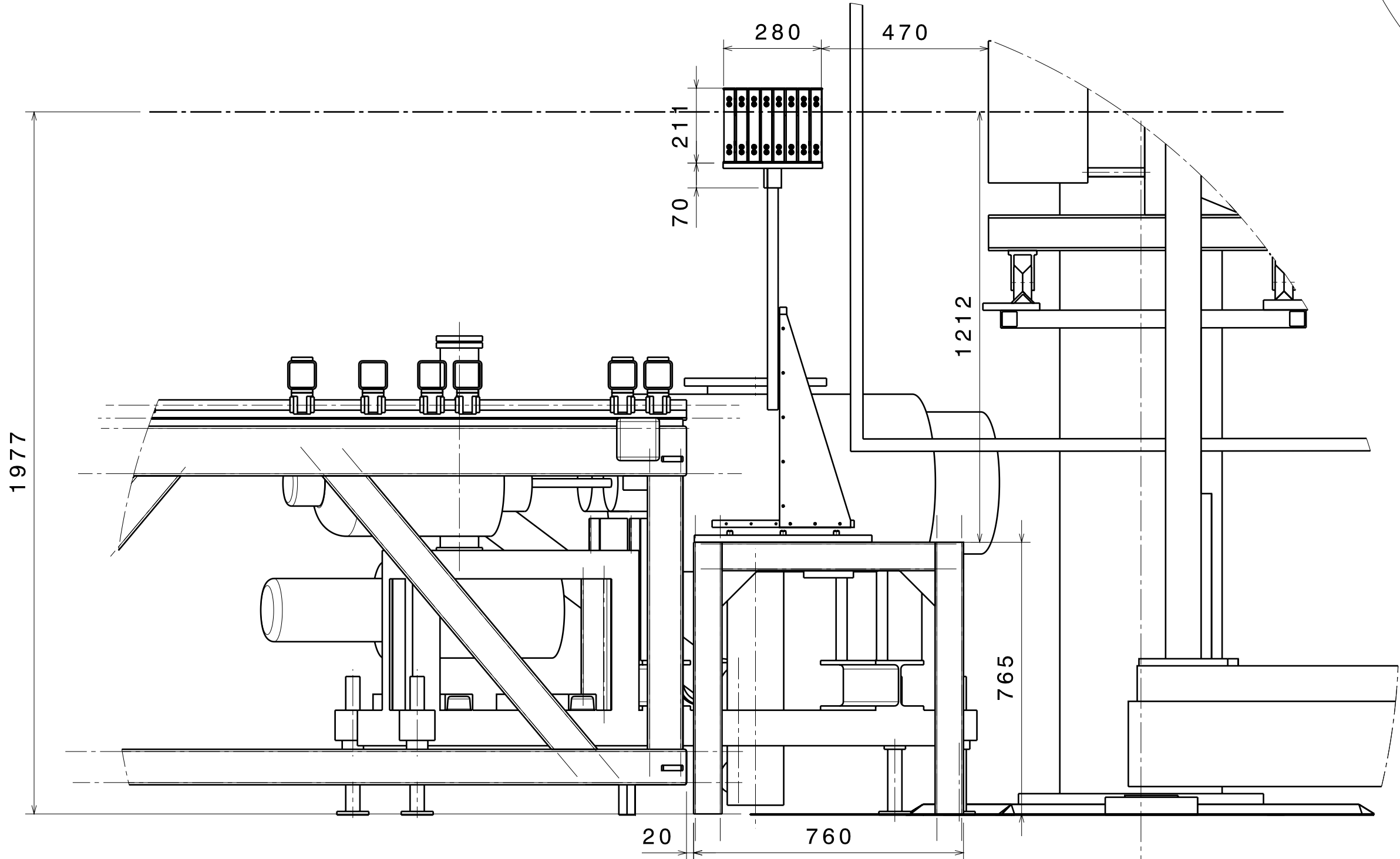
Détail A Echelle : 2:25
