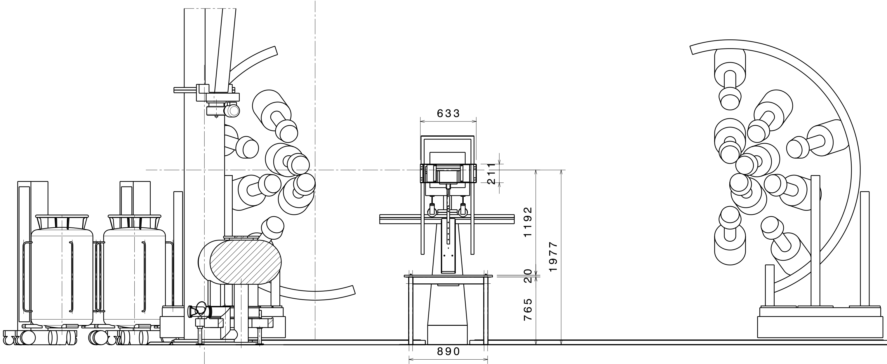
Coupe B-B Echelle : 1:25
